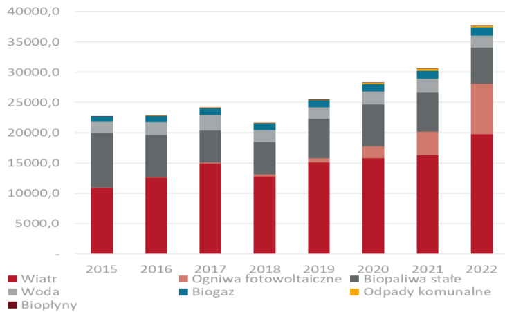
Produkcja energii z OZE w podziale na źródło (GWh)
