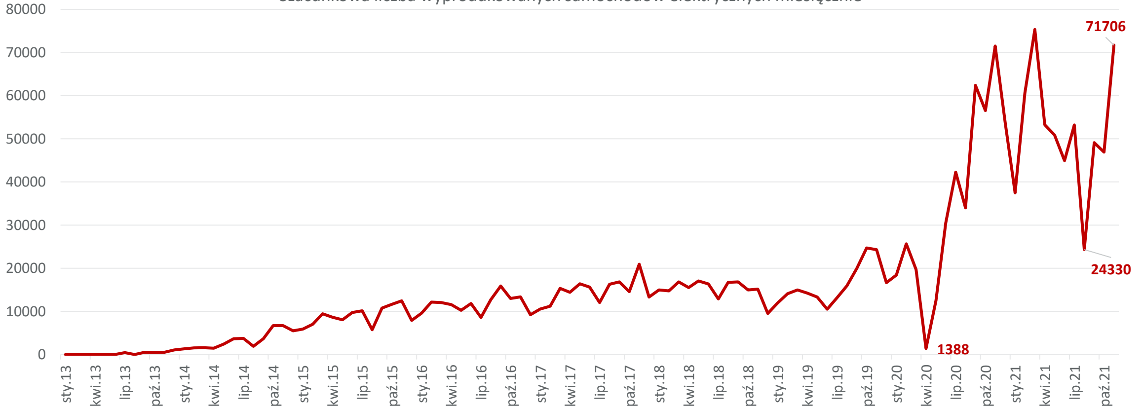
Szacunkowa liczba wyprodukowanych samochodów elektrycznych miesięcznie
