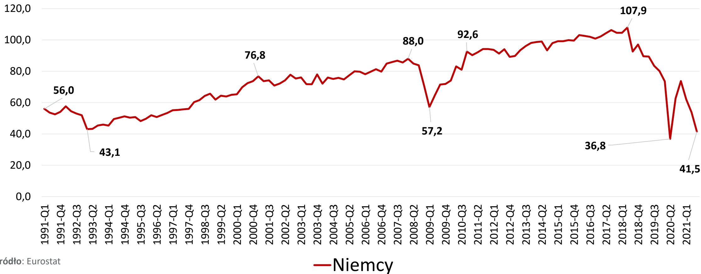
Produkcja pojazdów samochodowych, dane odsezonowane i pozbawione efektów kalendarzowych, indeks 2015=100
