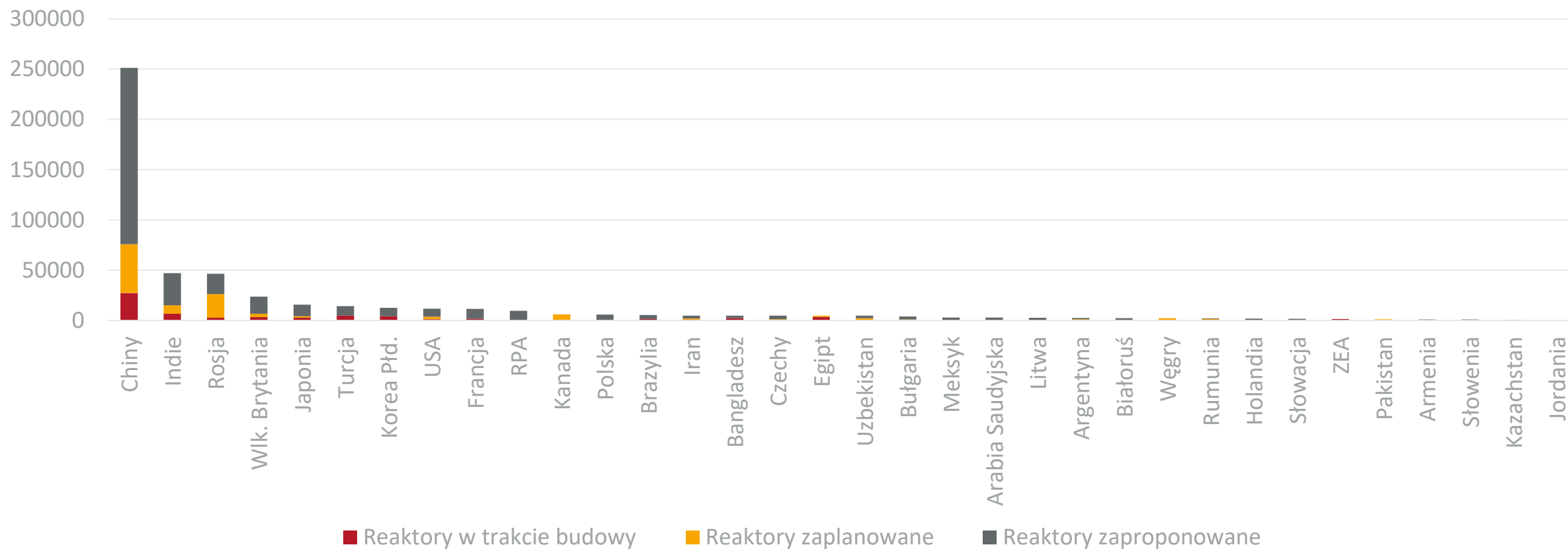
Moc budowanych, zaplanowanych i proponowanych reaktorów jądrowych (MWe, stan na sierpień 2023)
