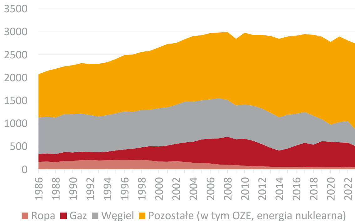
Produkcja energii elektrycznej w UE od 1985 r. w podziale na paliwo (TWh)
