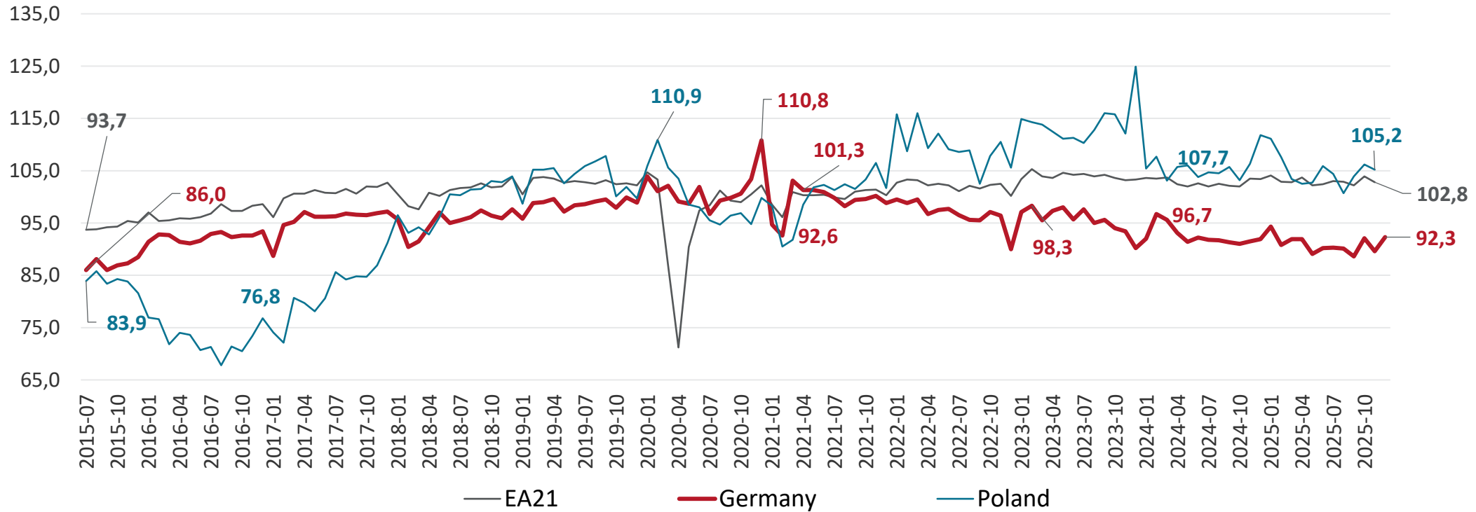
Budownictwo dane ogółem, indeks dane odsezonowane, pozbawione efektów kalendarzowych, indeks 2021=100
