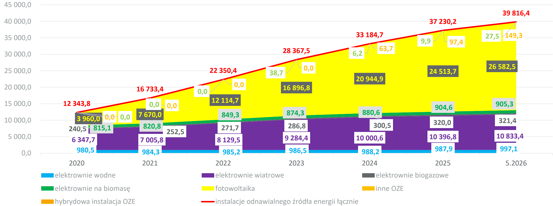
Rozwój mocy zainstalowanych w energetyce w Polsce w MW od 2020 r do maja 2026 r.
