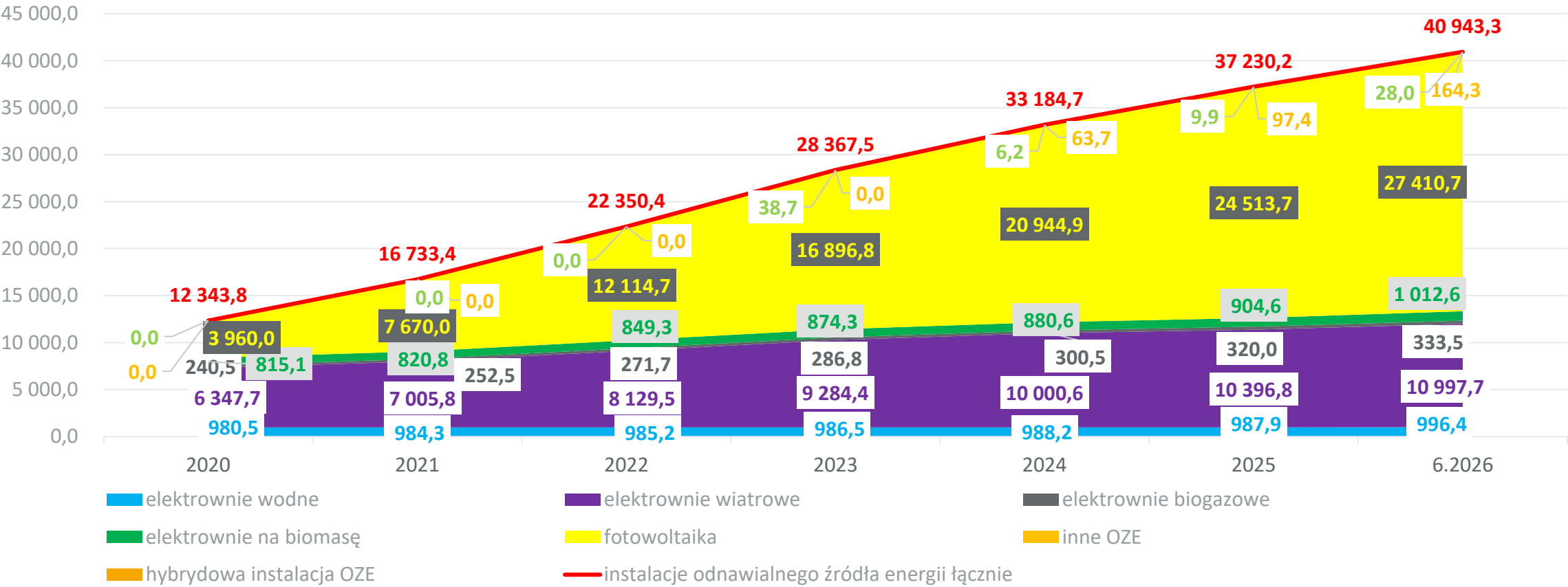
Rozwój mocy zainstalowanych w energetyce w Polsce w MW od 2020 r do czerwca 2026 r.
