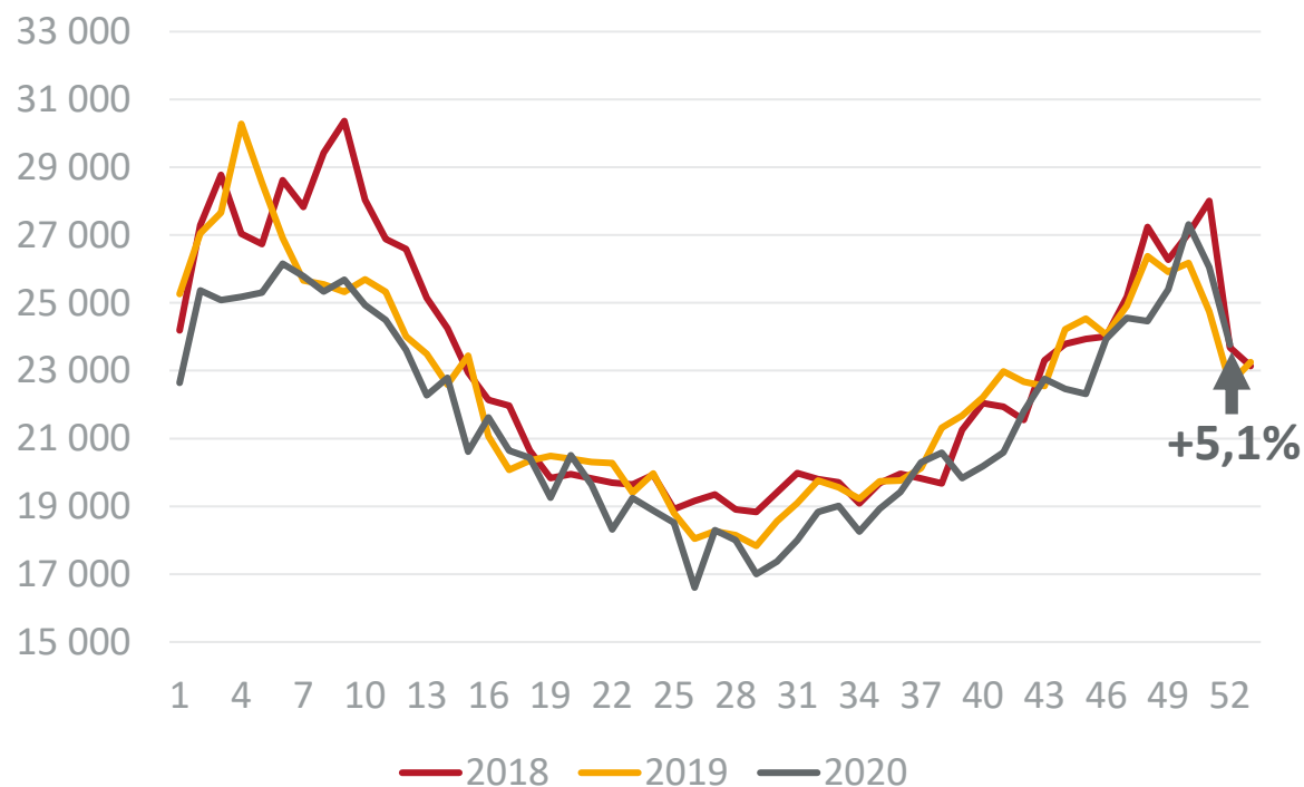
Średnie zapotrzebowanie na elektryczność (w MW) w Estonii w poszczególnych tygodniach roku
